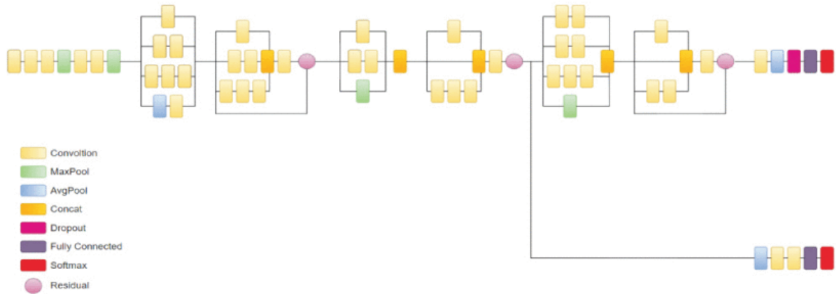
Şekil 1. InceptionResNetV2 mimarisi [4]
